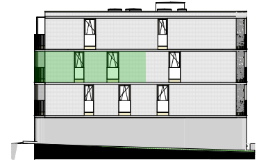
Zijgevel binnenplein
